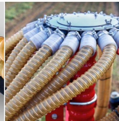
Düngeraufbau
