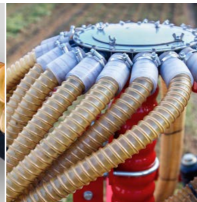
Düngeraufbau
