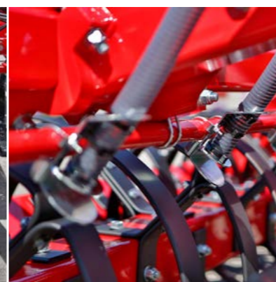
MiniDrill Saatgutverteiler legen das Saatgut direkt im feuchten Boden ab.
