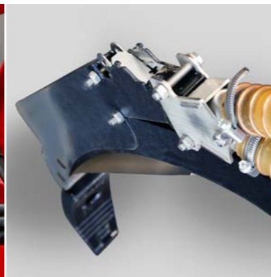
Düngerleitblech
